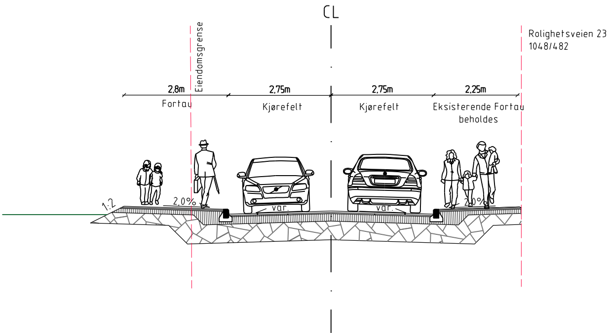
Normalprofil snitt C-C, Tors vei M=1:100 Vegmodell 10100 ca. pr.xx
