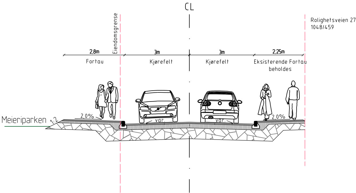
Normalprofil snitt B-B, G. Isevei M=1:100 Vegmodell 10200 ca. pr.xx
