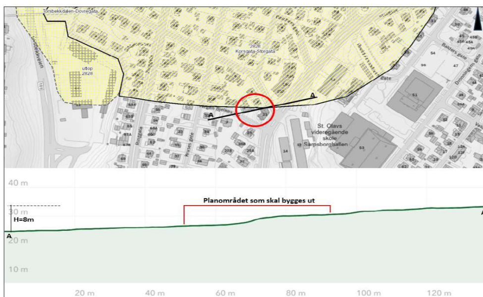
Bilde 2.2 Valg av kritisk snitt. Kilde: Rapport [1].
