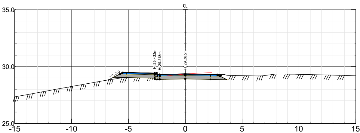
Kvastebyveien Pel nr 450 – Skala 1:200
