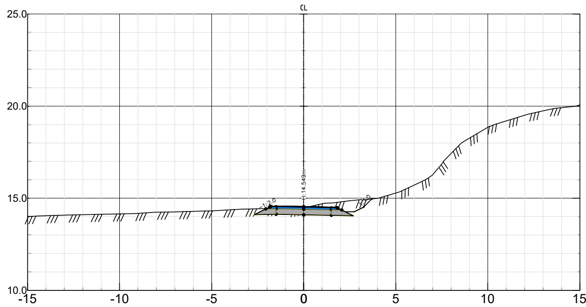
Gangvei Pel nr 200 – Skala 1:200
