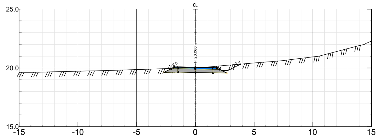
Gangvei Pel nr 300 – Skala 1:200
