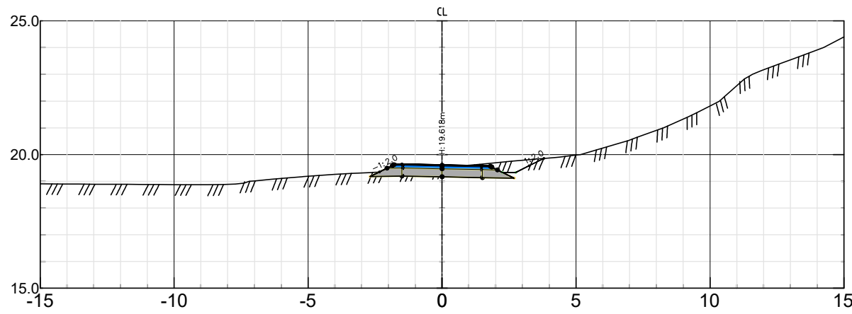
Gangvei Pel nr 330 – Skala 1:200
