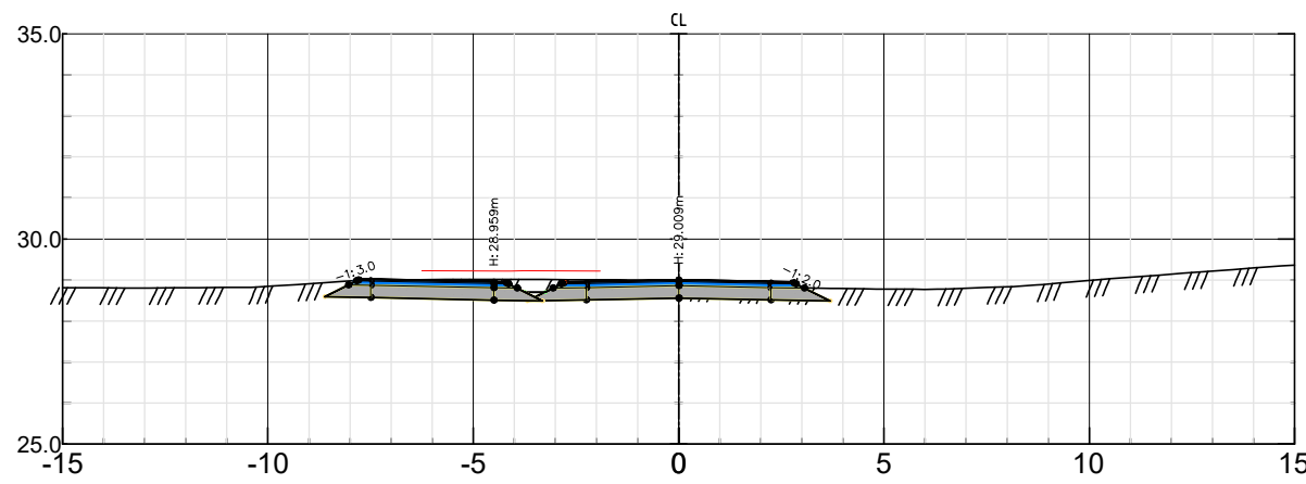
Kvastebyveien Pel nr 220 – Skala 1:200
