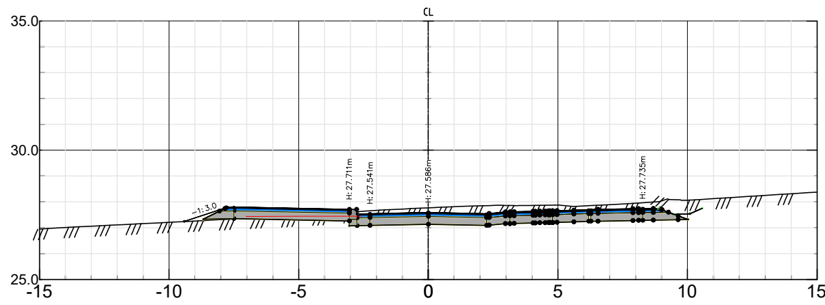
Kvastebyveien Pel nr 130 – Skala 1:200
