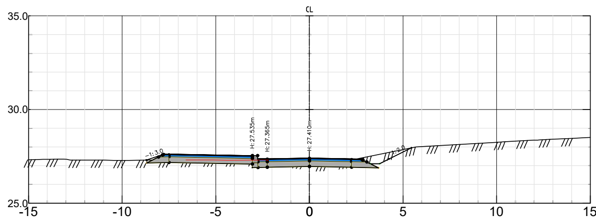
Kvastebyveien Pel nr 120 – Skala 1:200
