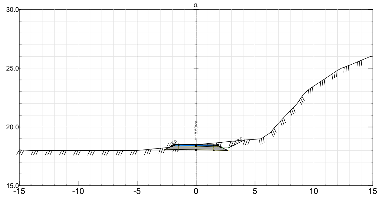
Gangvei Pel nr 360 – Skala 1:200
