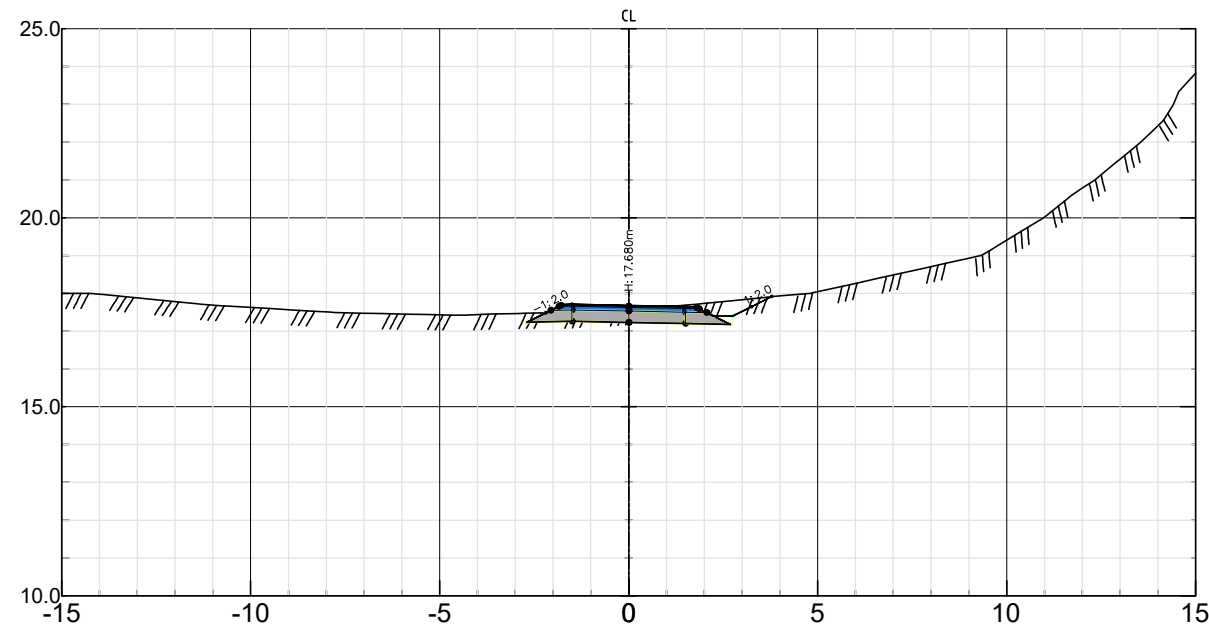
Gangvei Pel nr 380 – Skala 1:200
