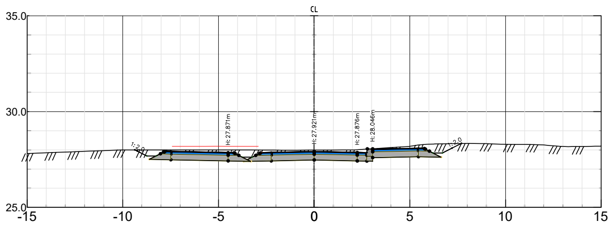
Kvastebyveien Pel nr 180 – Skala 1:200
