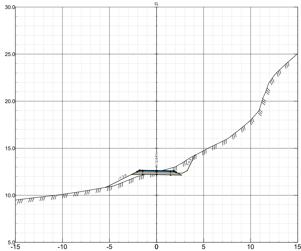
Gangvei Pel nr 530 – Skala 1:200
