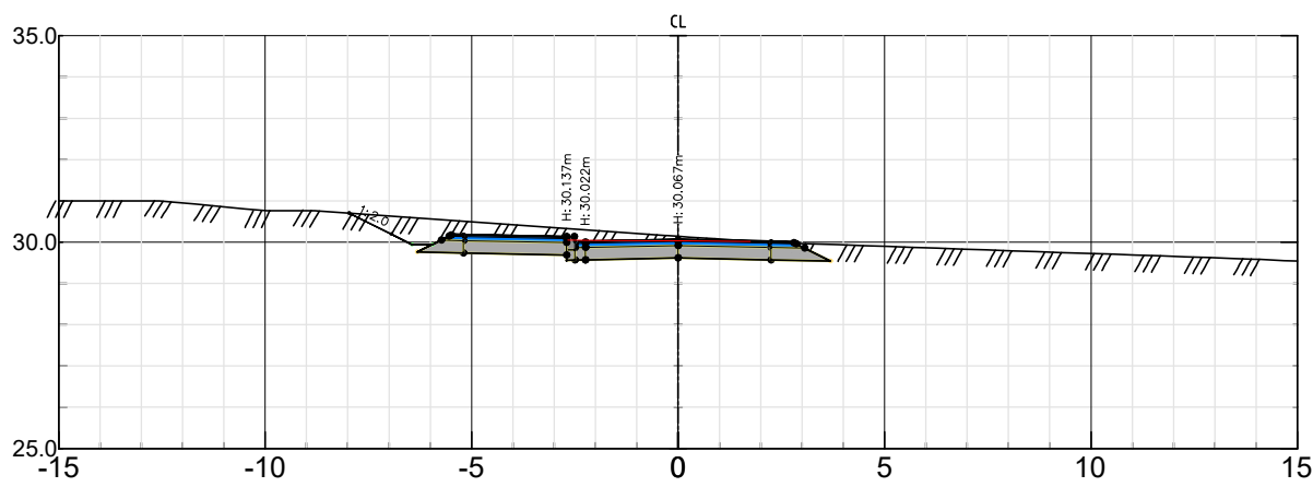
Kvastebyveien Pel nr 300 – Skala 1:200
