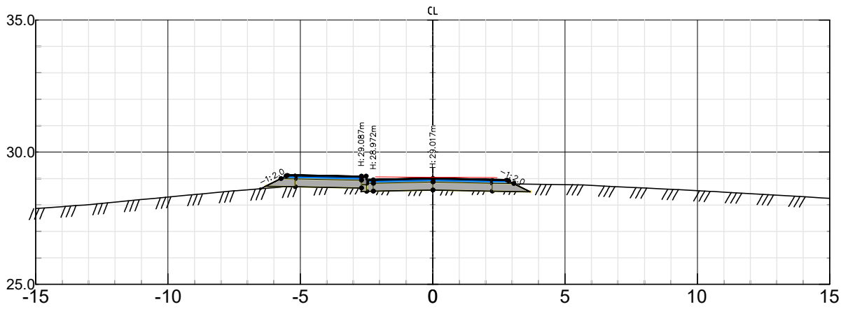
Kvastebyveien Pel nr 400 – Skala 1:200
