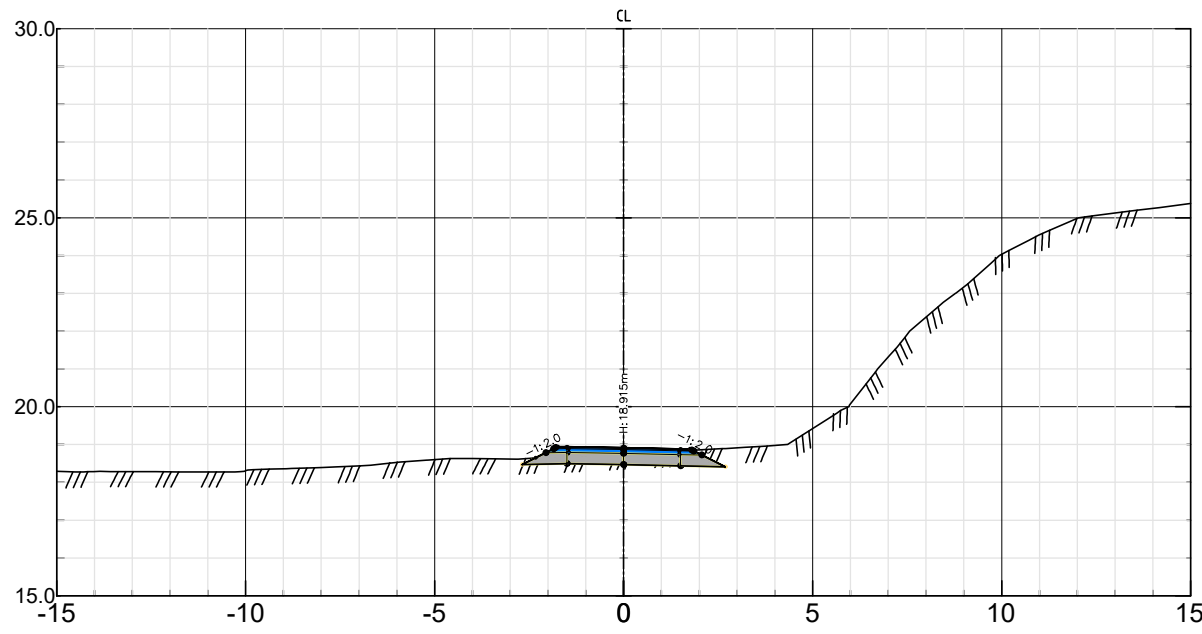
Gangvei Pel nr 350 – Skala 1:200
