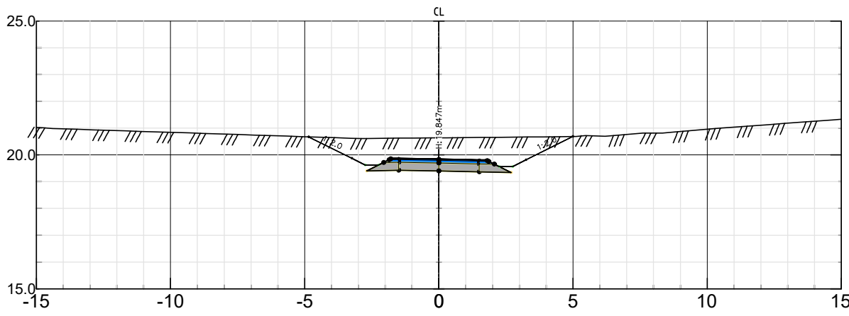
Gangvei Pel nr 260 – Skala 1:200
