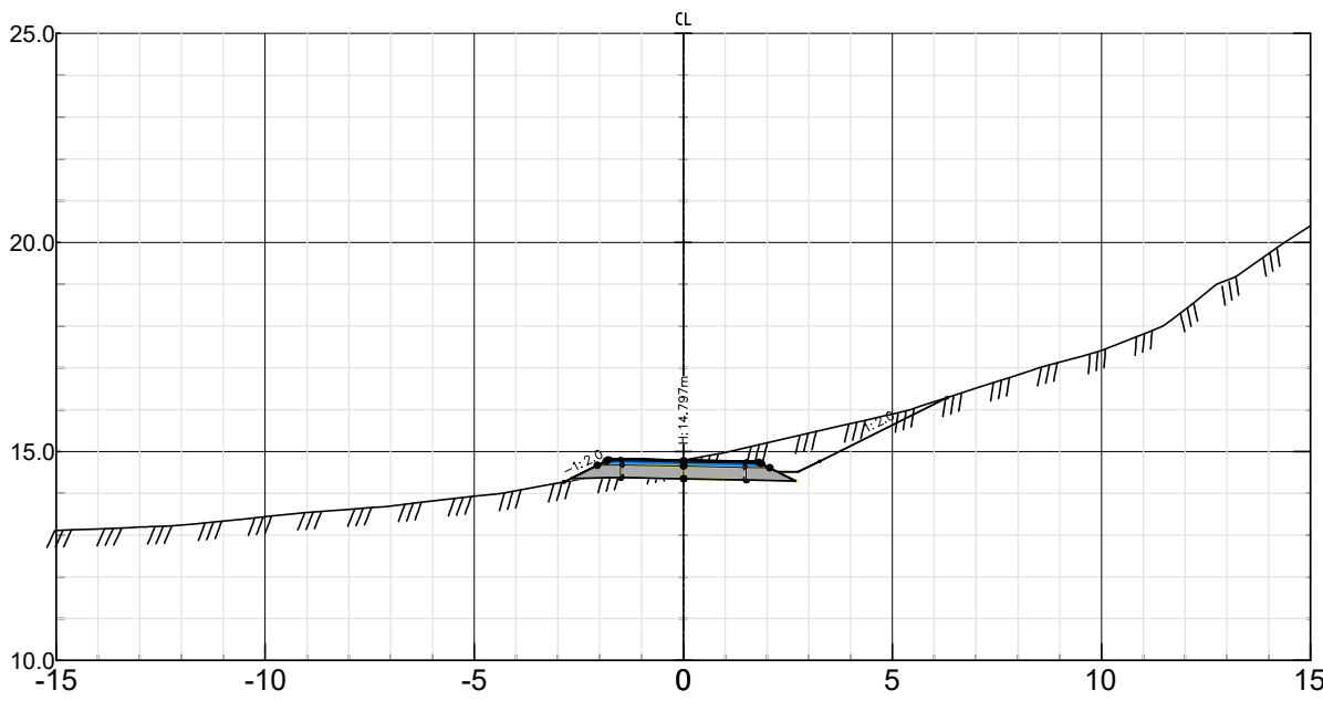
Gangvei Pel nr 470 – Skala 1:200
