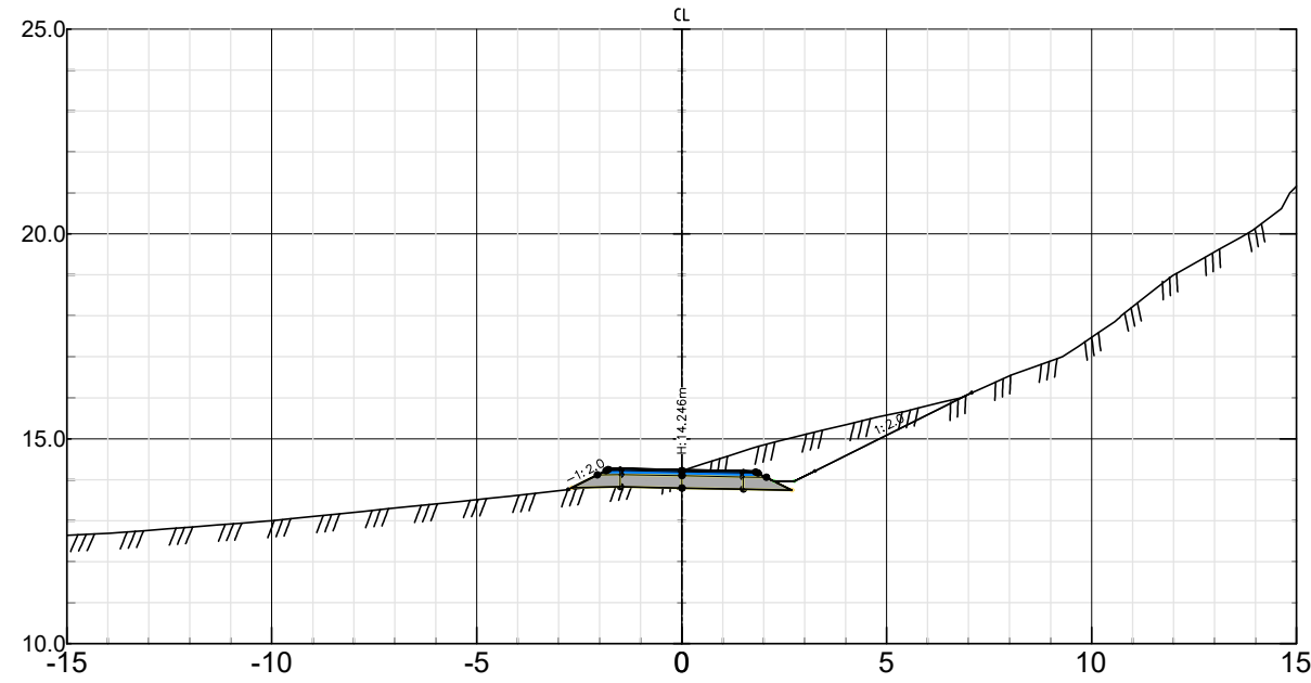
Gangvei Pel nr 480 – Skala 1:200
