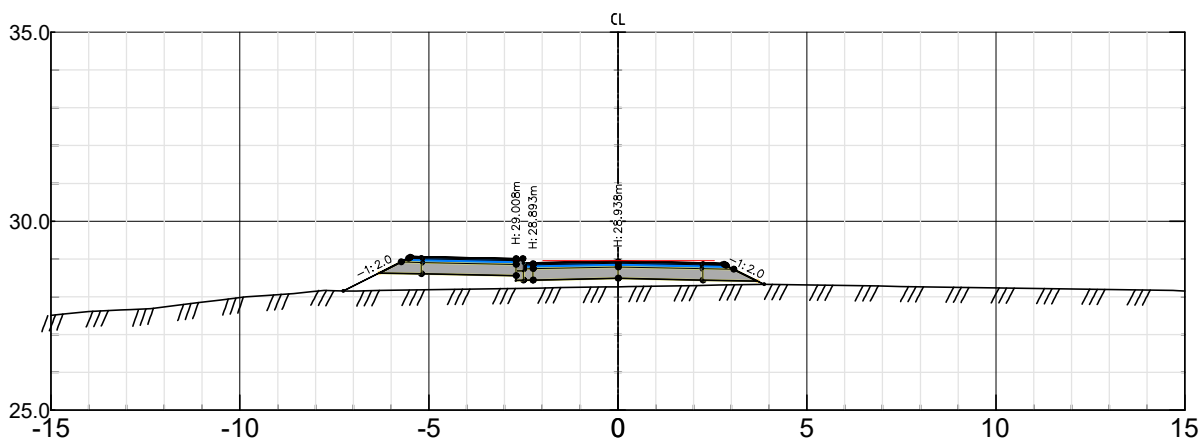
Kvastebyveien Pel nr 410 – Skala 1:200
