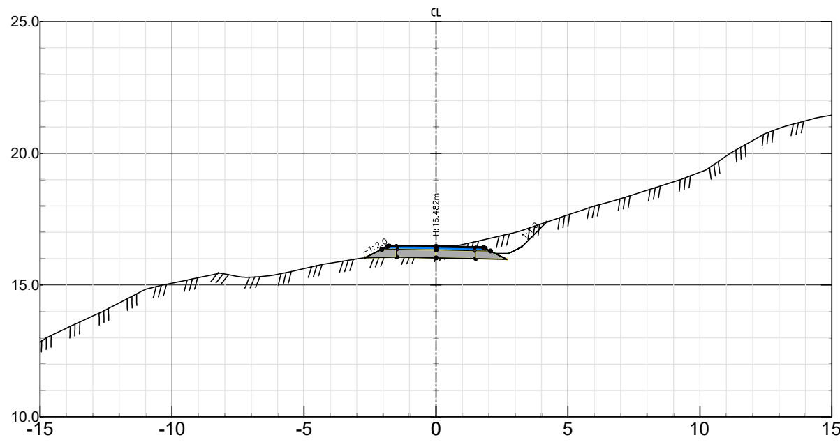
Gangvei Pel nr 680 – Skala 1:200
