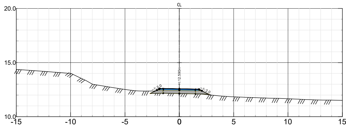
Gangvei Pel nr 180 – Skala 1:200
