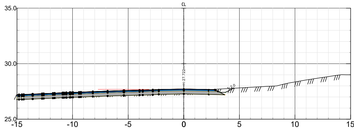
Kvastebyveien Pel nr 150 – Skala 1:200
